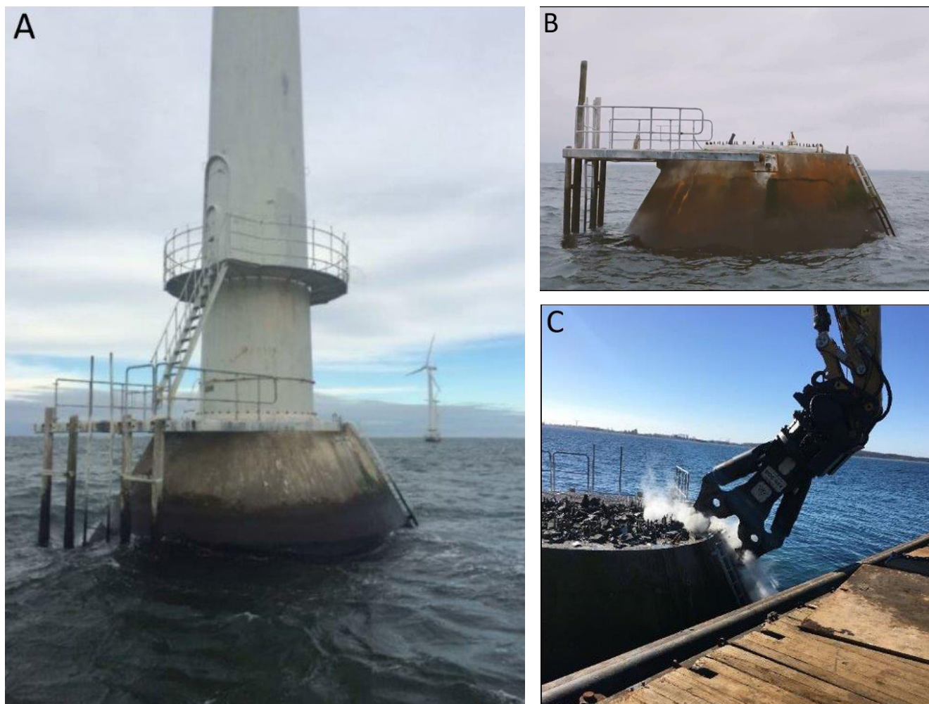
Figur 2. Fjernelse af verdens første havvindmølle park, der stod ved Vindeby på Lolland i perioden 1991 – 2017. Fundamenterne rummede ingen miljøfarlige stoffer /9/. Hvert fundament var et gravitationsfundament og havde en top-diameter på 5 m og en bund-diameter på 14 m. Fundamenterne blev bl.a. fjernet med en hydraulisk betonsaks. Fjernelsen af fundamenterne kostede ifølge Ørsted A/S et mindre tocifret millionbeløb. Billede A er fra /9/ og B og C er taget af Ørsted A/S.
